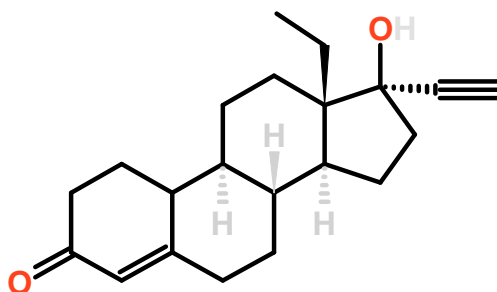
Levonorgestrel
